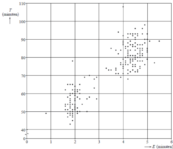
Figuur 4. Eruptietijden en tussentijden van Old Faithful
