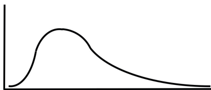
Figuur 2. Scheve verdeling.
