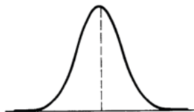
Figuur 1. Normale verdeling.
