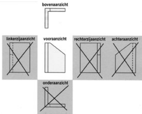
fig. 4 De aanzichten van het hoekprofiel. Doorgestreepte aanzichten bevatten overbodige informatie
