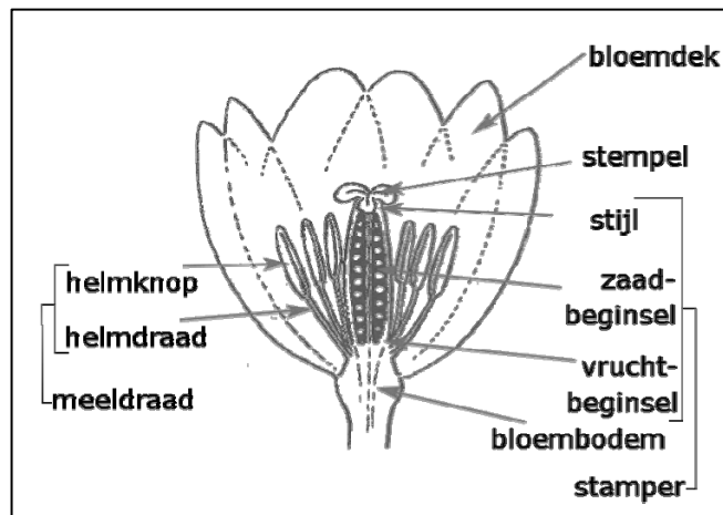
Figuur 1: De stamper van een plant vlak voor bevruchting (aangepast uit Kersbergen, Carla, & Haarhuis, Amito, 2002. Natuuronderwijs Inzichtelijk . Bussum: Uitgeverij Coutinho, p. 56)
