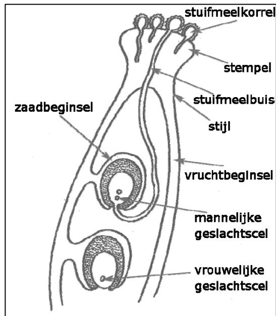
Figuur 2: Overzicht van de onderdelen van een bloem die een rol spelen bij de geslachtelijke voortplanting (aangepast uit Kersbergen, Carla, & Haerhuis, Amito, 2002. Natuuronderwijs Inzichtelijk . Bussum: Uitgeverij Coutinho, p. 50)
